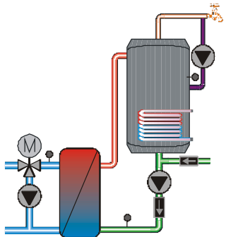
WW SLS-Prim.Par.
