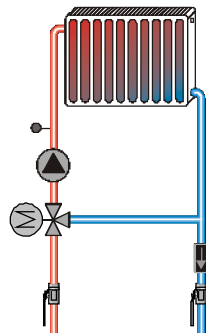
Gemischter Heizkreis
