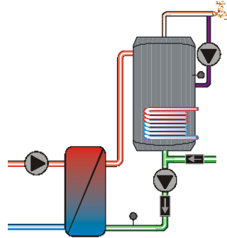
WW SLS-Sekundär
